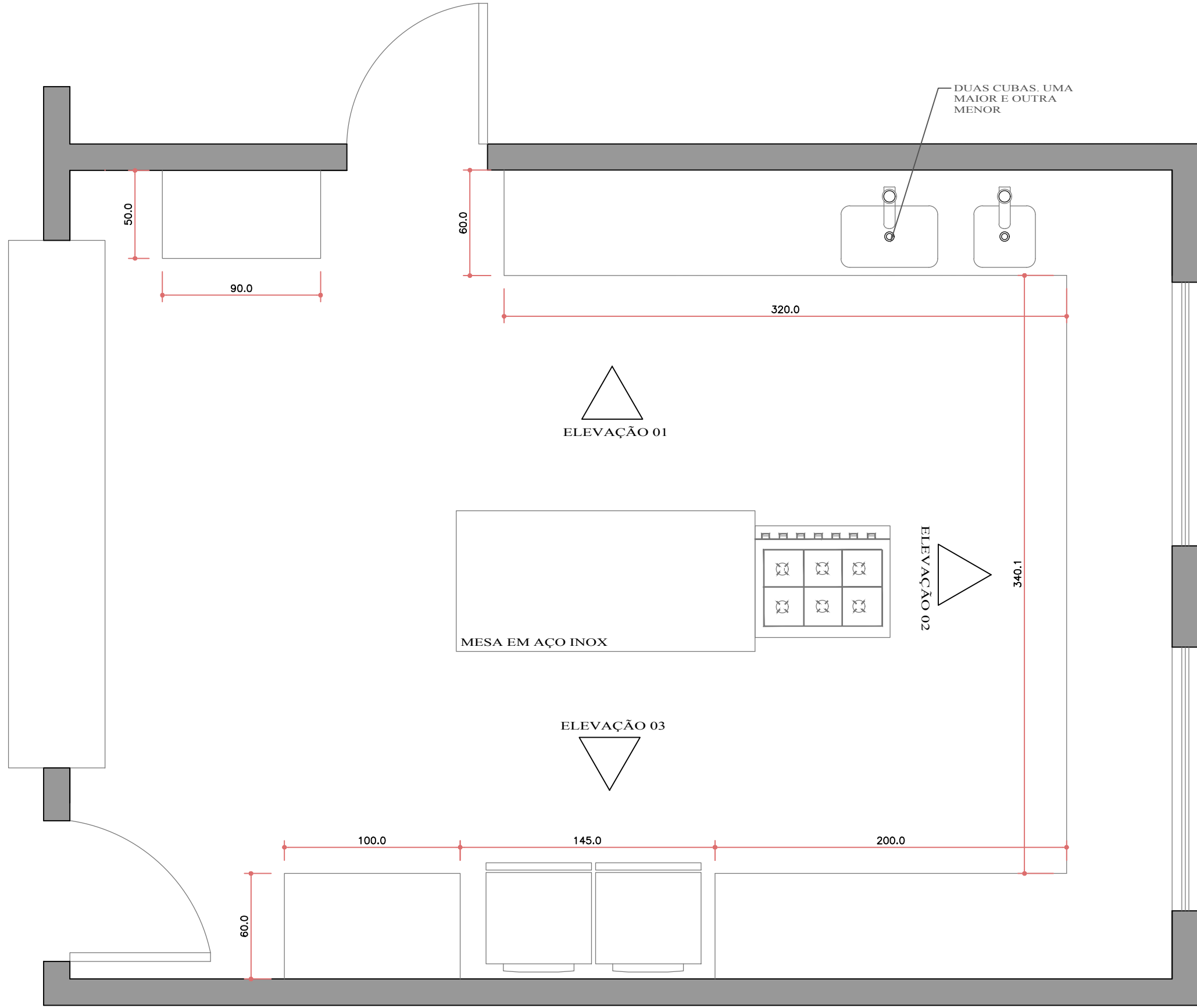
PLANTA BAIXA COZINHA ESCALA: 1/25
