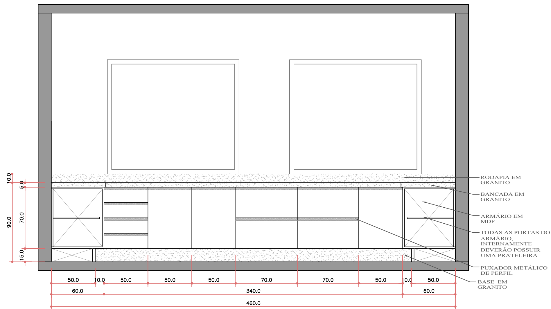
ELEVAÇÃO 02 ESCALA: 1/25
