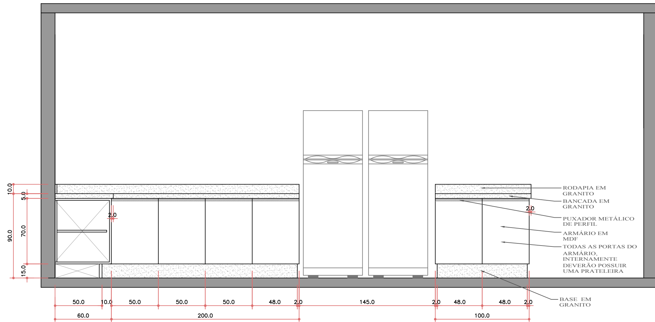
ELEVAÇÃO 03 ESCALA: 1/25
