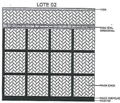
MEIO DE QUADRA LOTE 02 ESCALA: 1/50
