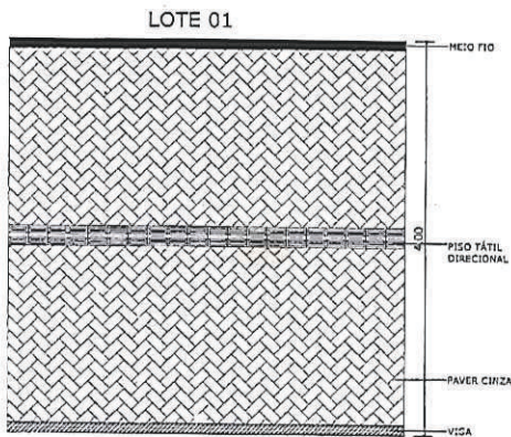
MEIO DE QUADRA LOTE 01 ESCALA: 1/50
