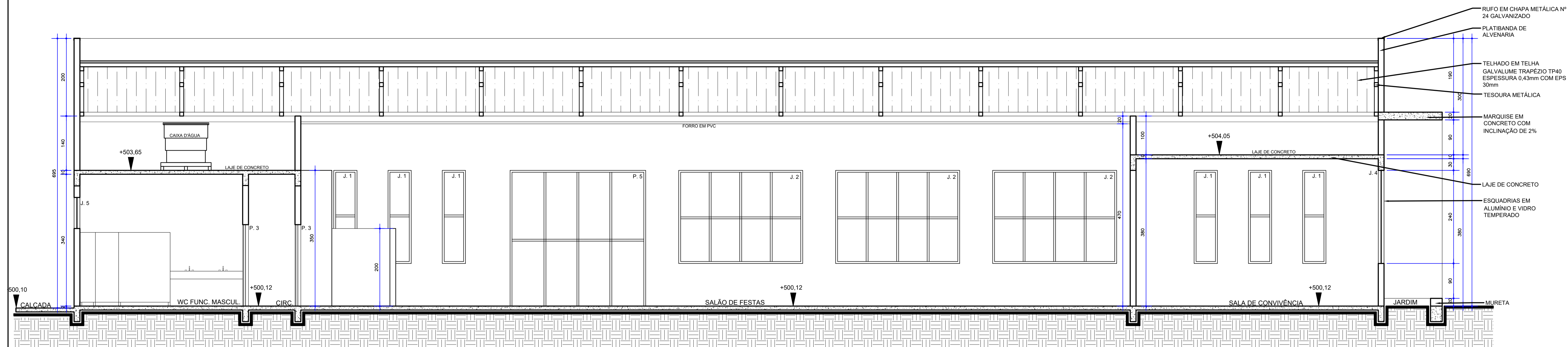
CORTE B ESCALA: 1/50
