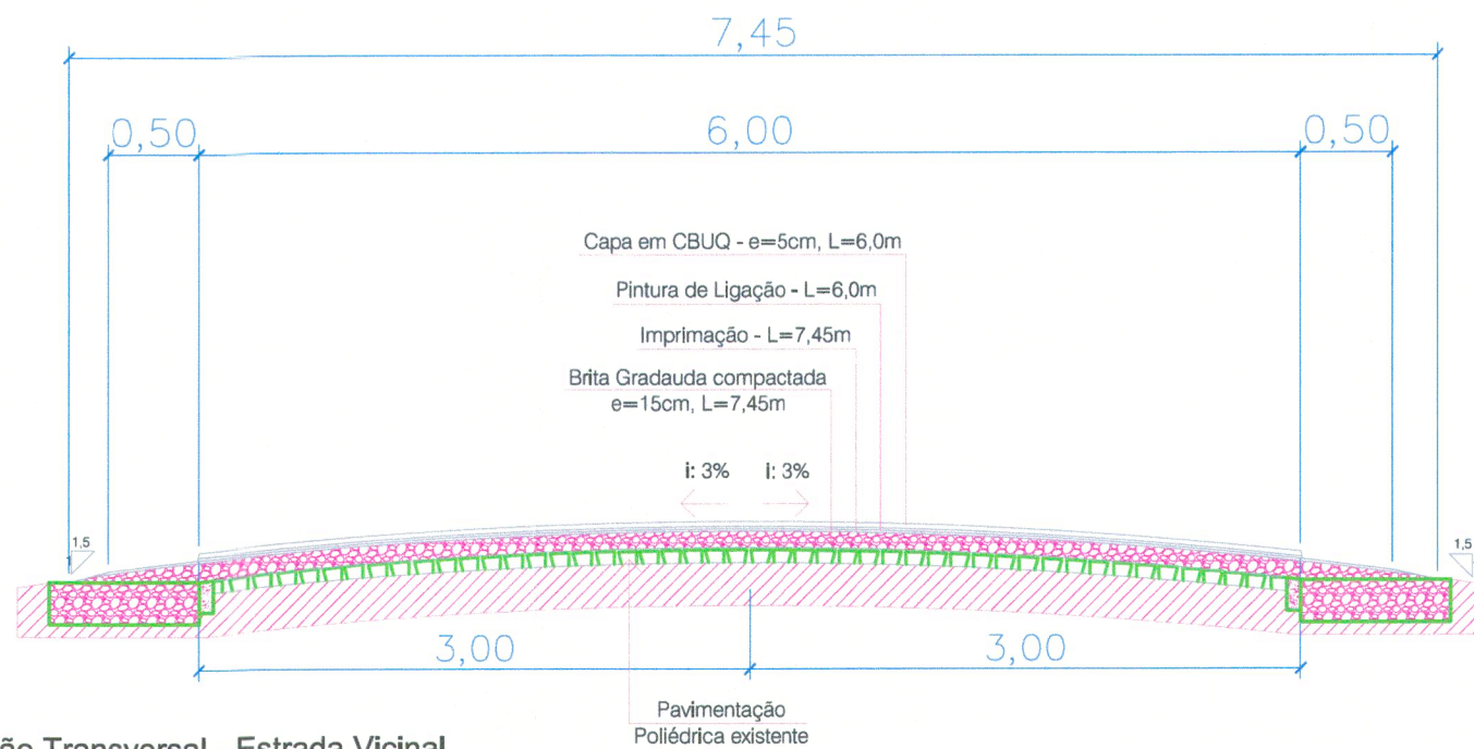
Seção Transversal - Estrada Vicinal Extensão: 5.100m Área: 30.600,00m 2
