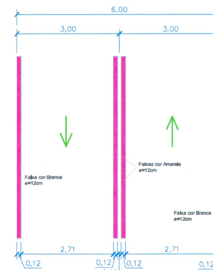
Detalhe das faixas Horizontal Delimitação de Vias S/Escala
