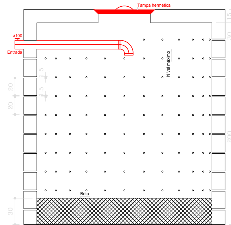
SUMIDOURO CORTE - ESC. 1:25
