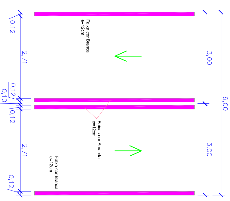
Detalhe das faixas Horizontal Delimitação de Vias S/Escala
