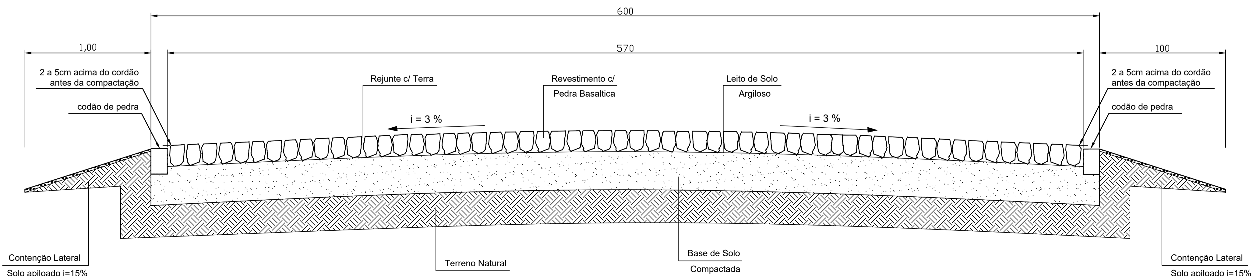
Perfil Longitudinal Escala: 1:20
