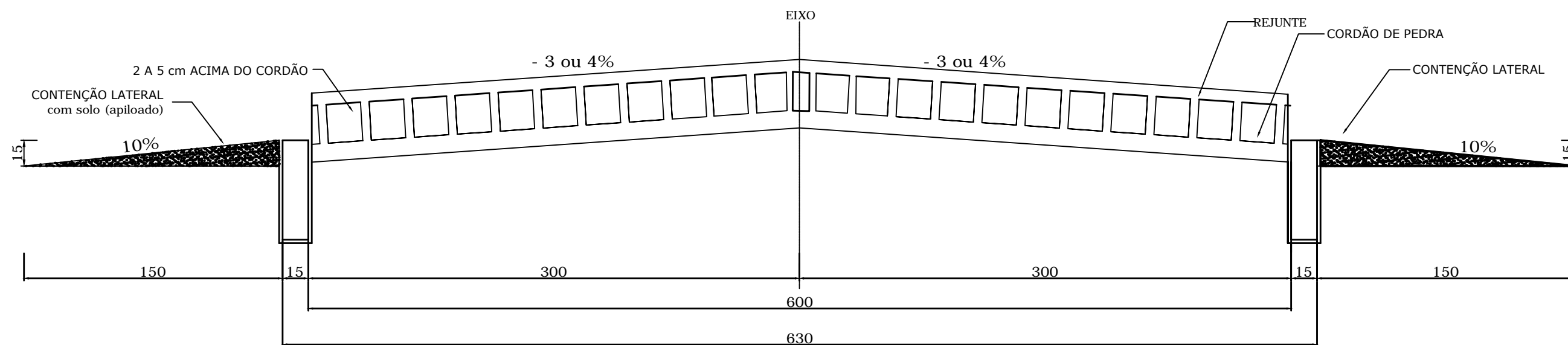
Perfil Longitudinal Escala: 1:25
