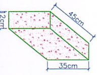
Dimensões Mínimas do Cordão de Pedra
