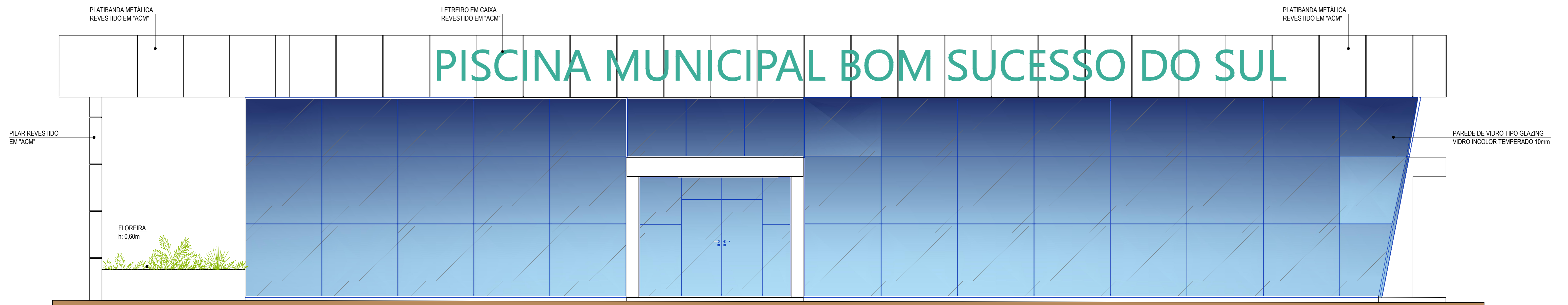
Elevação Frontal Escala= 1 : 50
