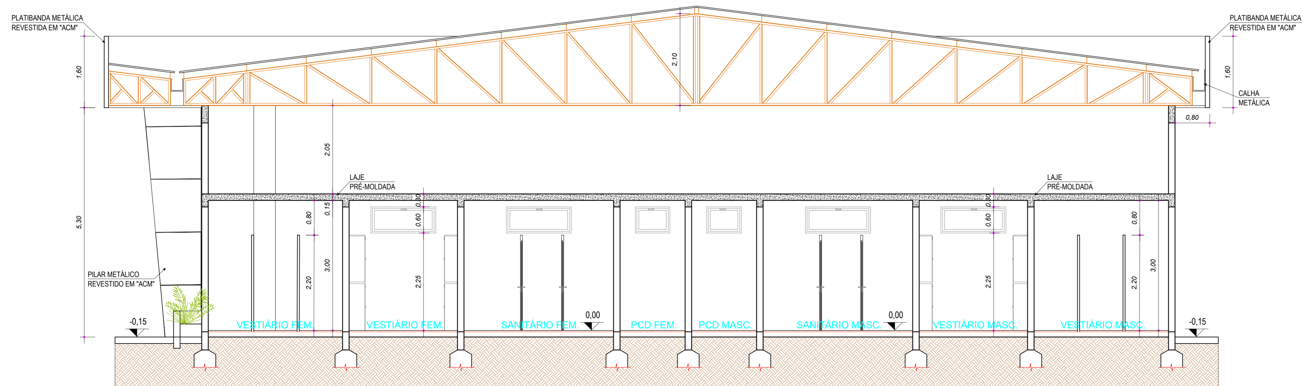
Corte C - C (Transversal) Escala= 1 : 50
