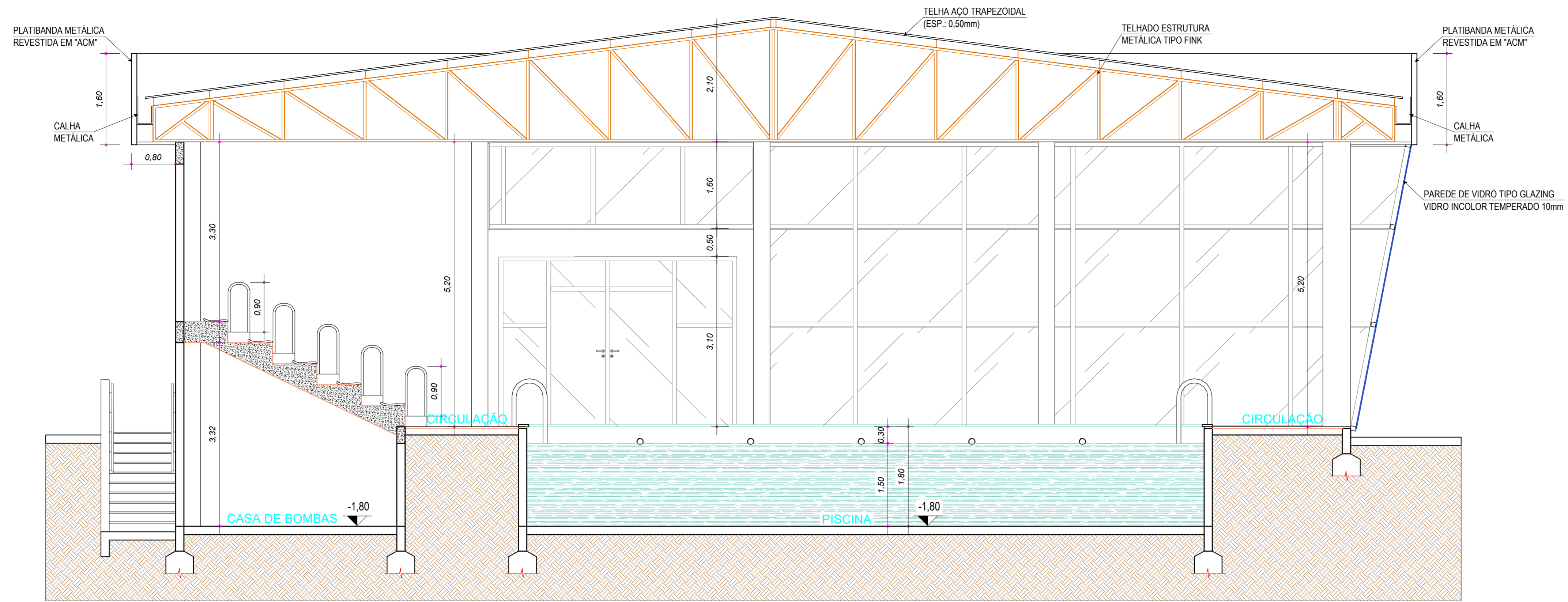
Corte D - D (Transversal) Escala= 1 : 50
