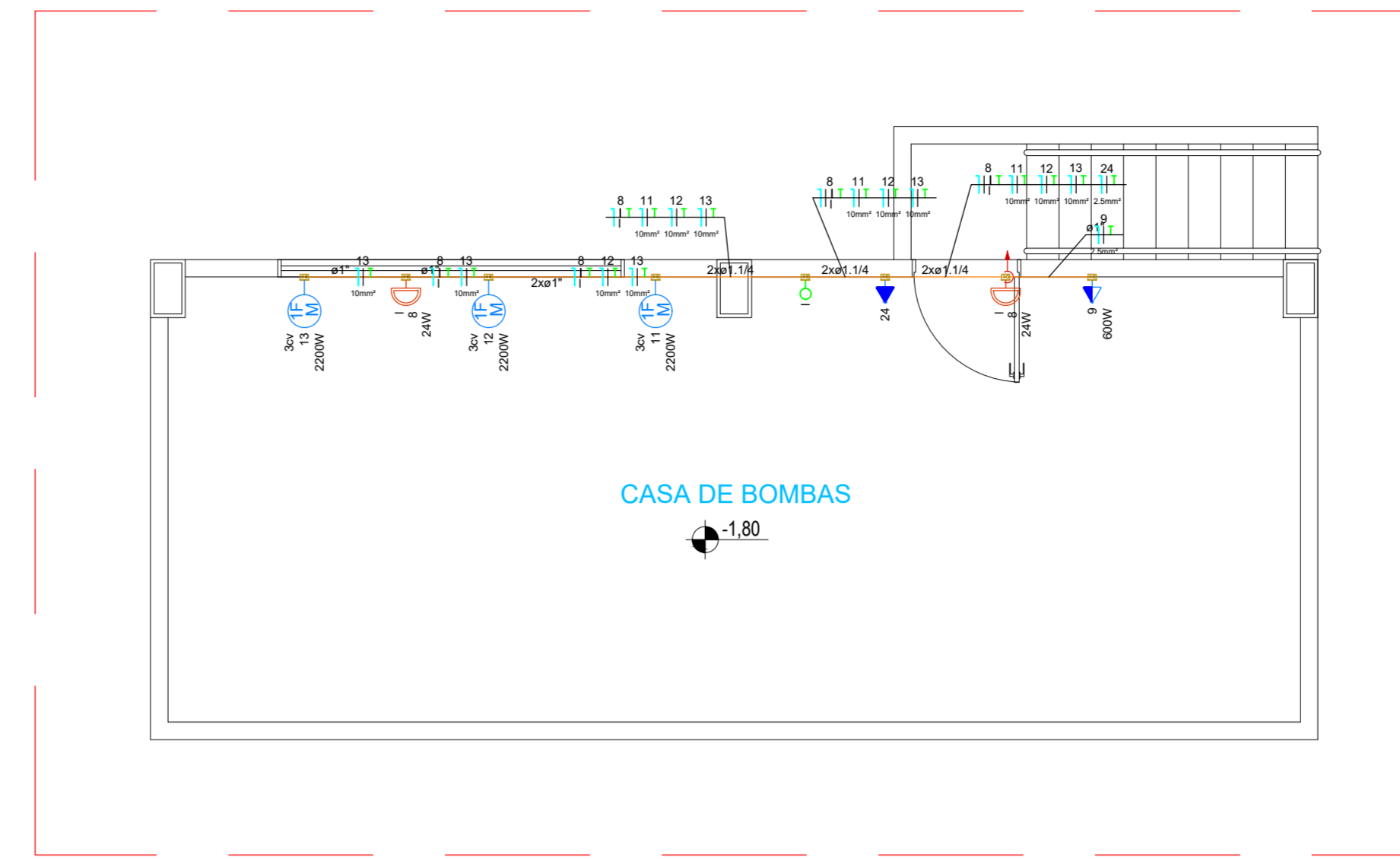
Planta Baixa Pav.Sub-Solo Escala= 1 : 50
