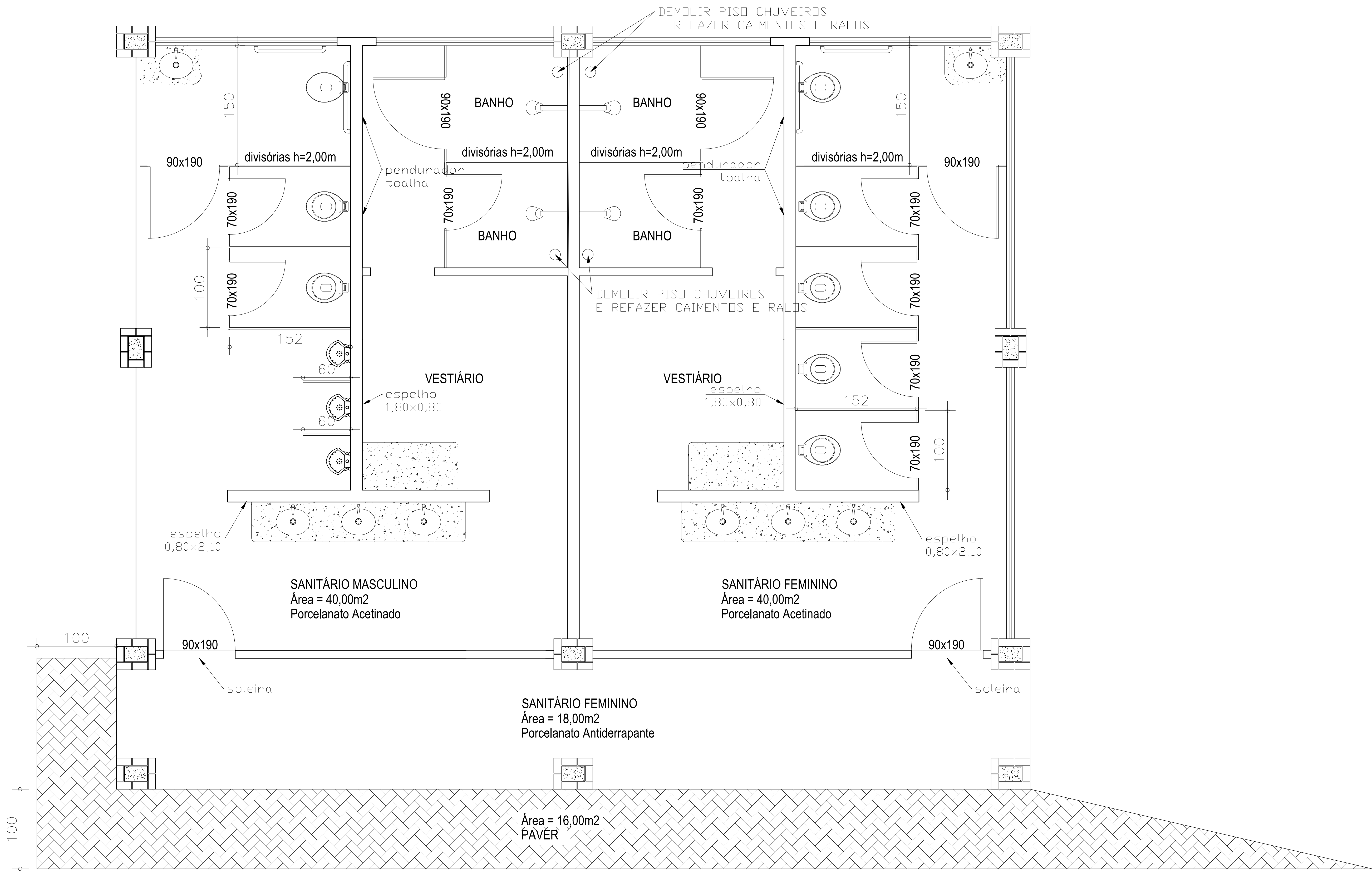
LAYOUT REFORMA BANHEIROS ÁREA=98,00m2
