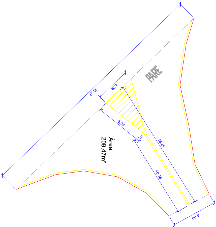
Projeto Geométrico - Detalhe 2
