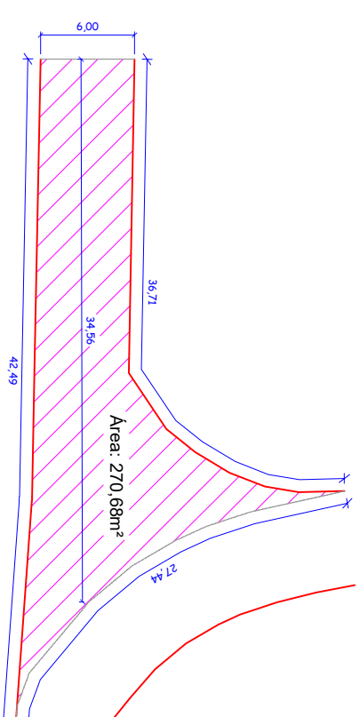
Projeto Geométrico - Entroncamento 4 S/Escala
