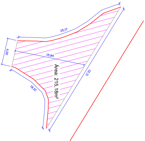
Projeto Geométrico - Entroncamento 1 S/Escala
