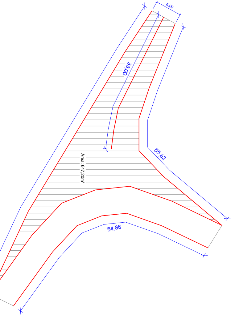
Projeto Geométrico - Entroncamento 2
