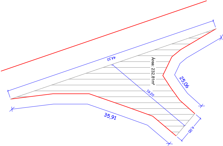
Projeto Geométrico - Entroncamento 1
